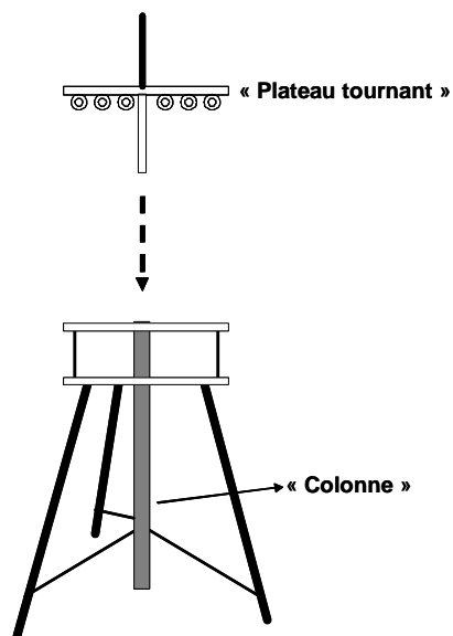
Figure 17 Axe du plateau tournant dans la colonne
